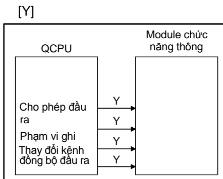
Hình 7.4 Tín hiệu Y của CPU
