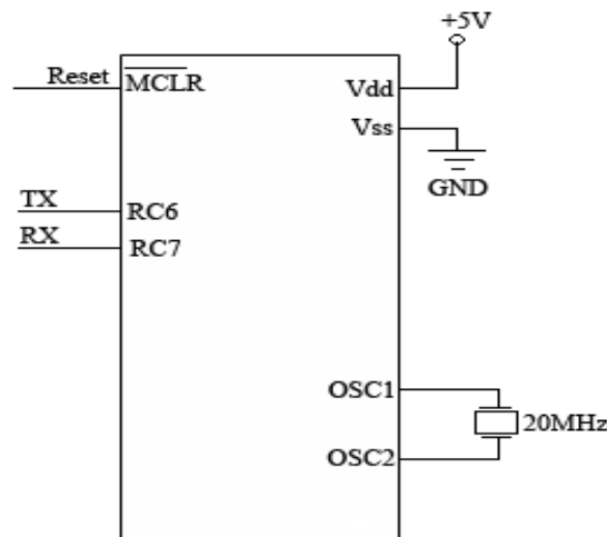
Hình 2-43. Các đường giao tiếp với mạch nạp nối tiếp qua IC chuyển đổi.
