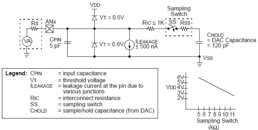
Hình 2-23. Sơ đồ mạch của ngõ vào ADC.
