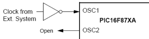
Hình 2-32. Ngõ vào nhận xung từ bên ngoài cấu hình XT, LP hoặc HS.
