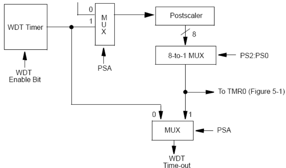
Hình 2-39. Sơ đồ khối của WDT.
