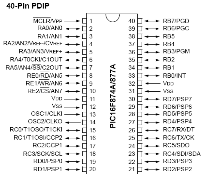
Hình 2-3. Sơ đồ chân
