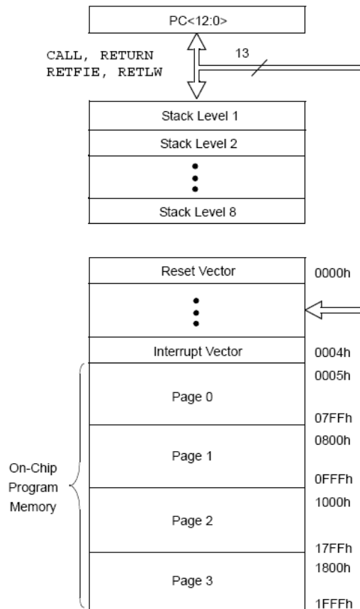
Hình 2-4. Sơ đồ bộ nhớ chương trình và ngăn xếp.
