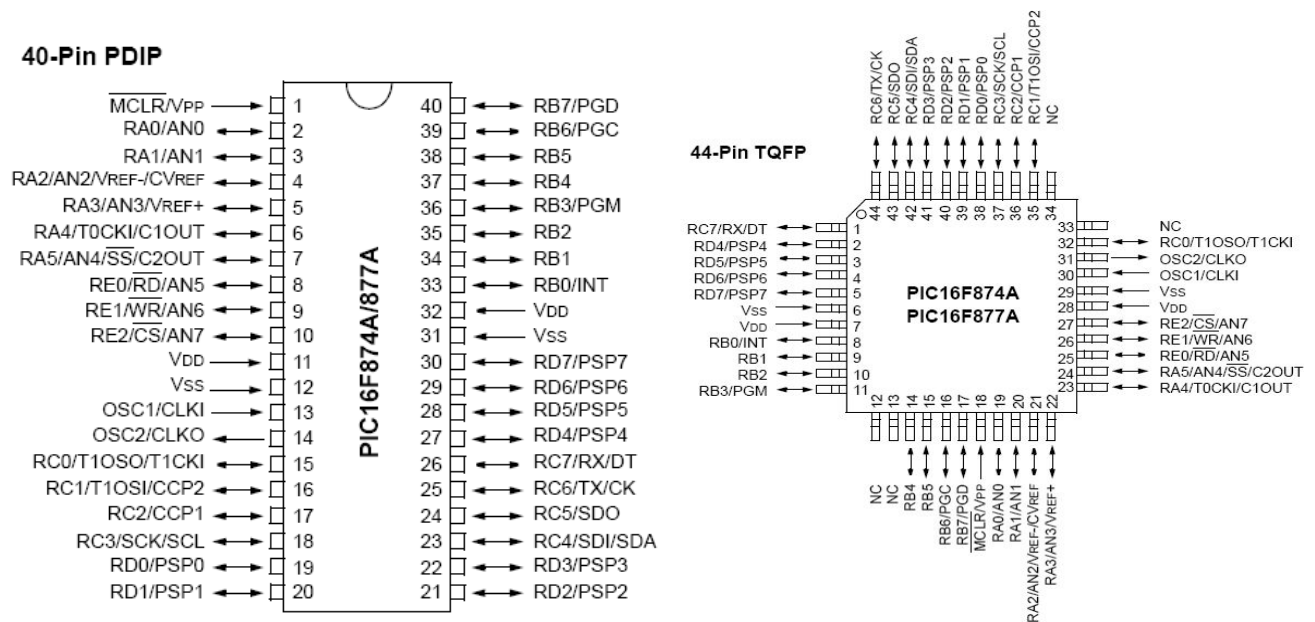
Hình 2-1. Sơ đồ chân họ PIC16F87XA.
