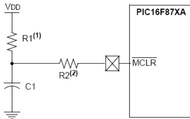
Hình 2-34. Mạch reset.
