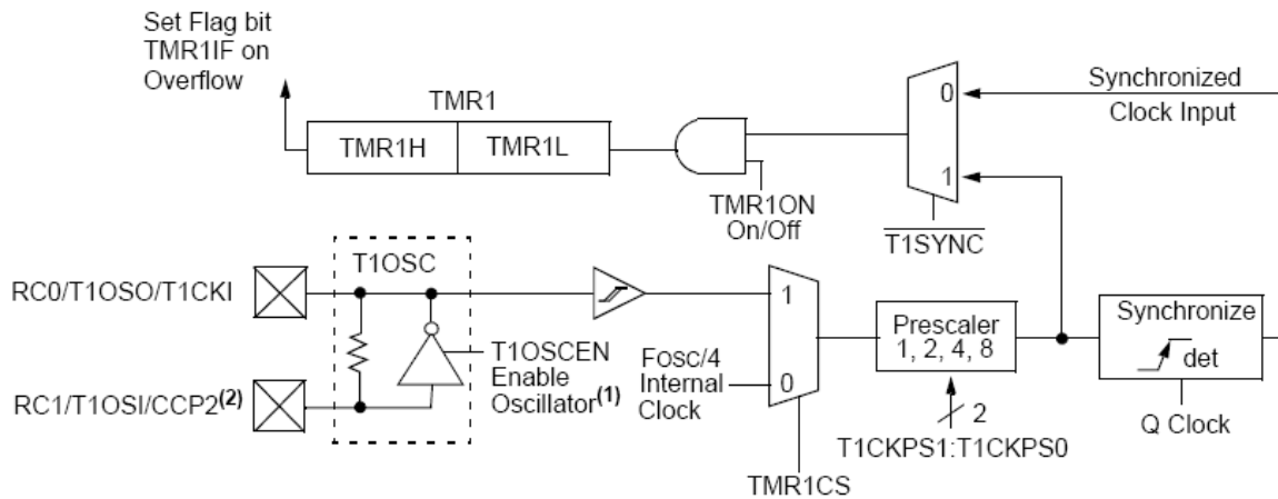
Hình 2-20. Sơ đồ khối của Timer1.
