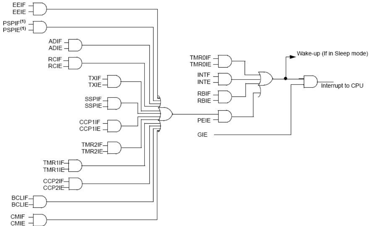
Hình 2-38. Sơ đồ logic của các ngắt.
