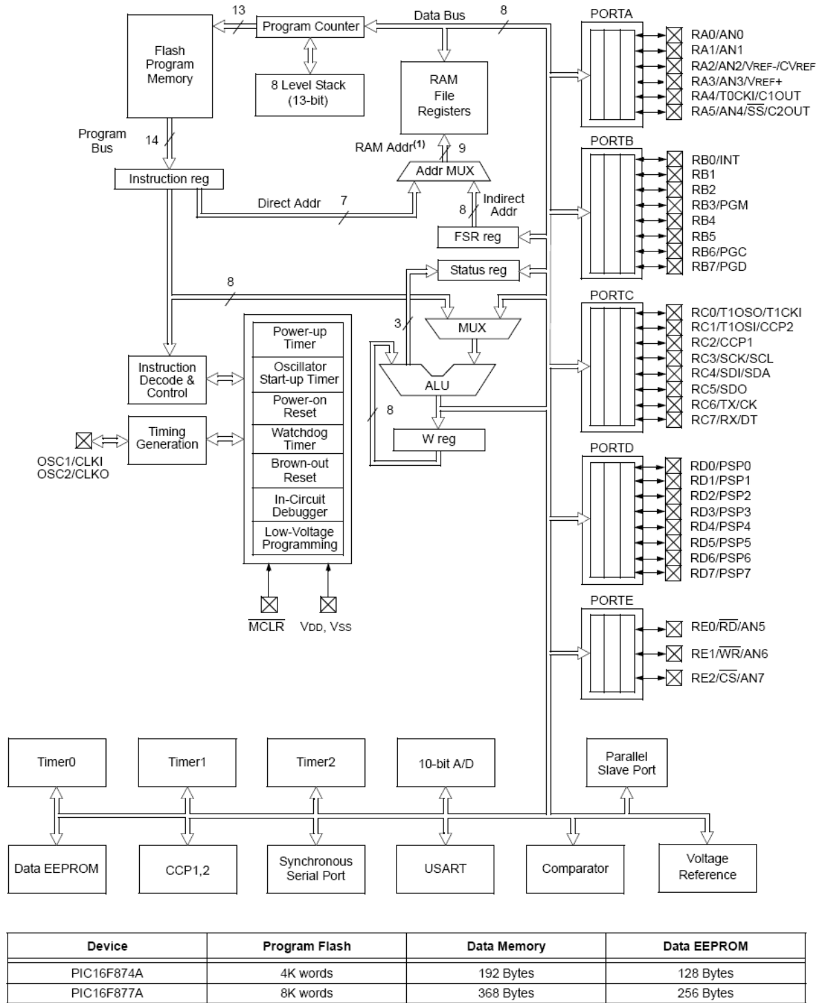
Hình 2-2. Sơ đồ khối PIC16F87XA.
