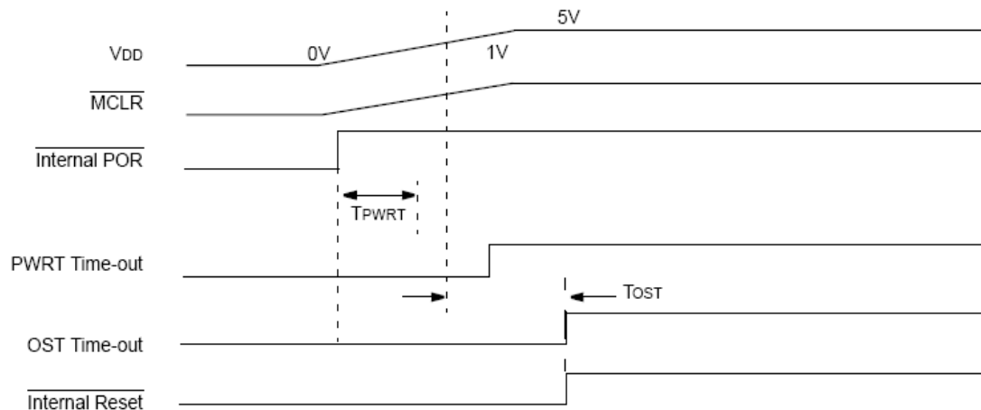
Hình 2-37. Trình tự thời gian khi reset POR không nối \overline{MCLR} .
