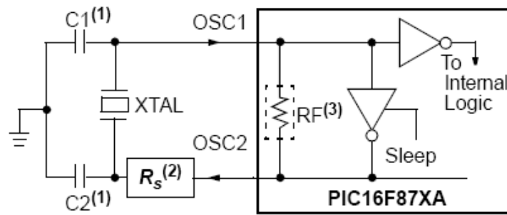
Hình 2-31. Dao động dùng thạch anh/tụ cộng hưởng cấu hình XT, LP hoặc HS.
