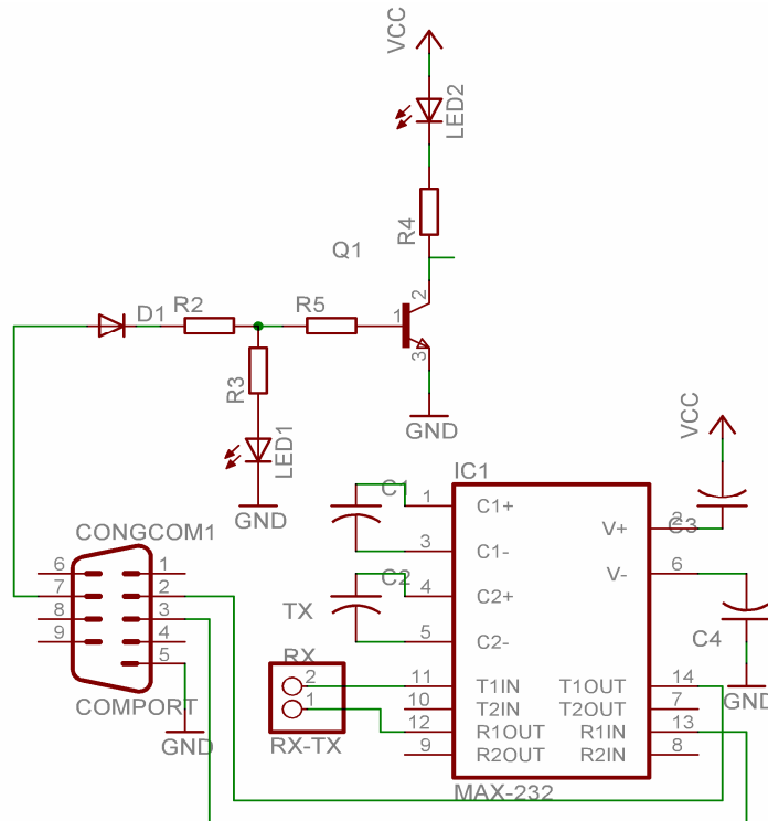
Hình 2-44. Sơ đồ nguyên lý mạch nạp nối tiếp từ cổng COM qua IC chuyển đổi.
