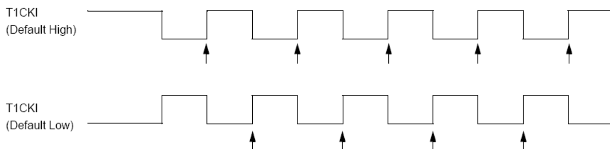
Hình 2-19. Giảm đồ thời gian xung đếm của Counter1.
