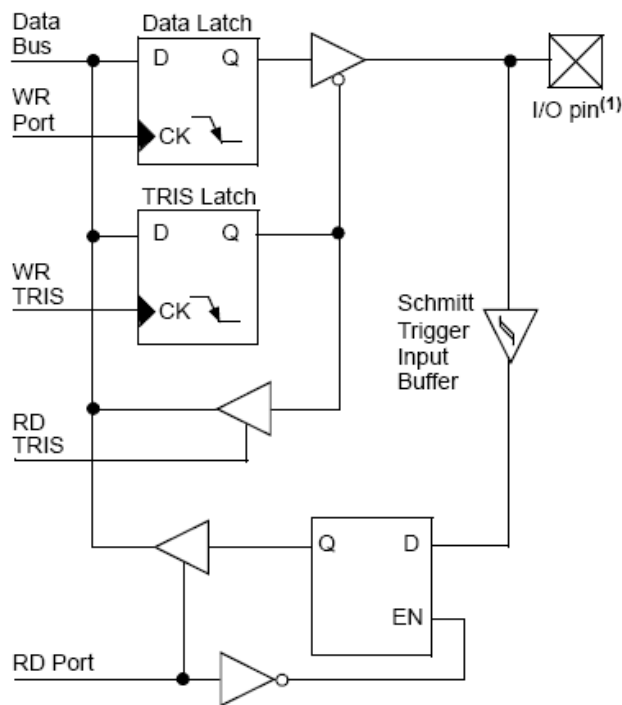
Hình 2-17. Sơ đồ mạch các chân PORTE.
